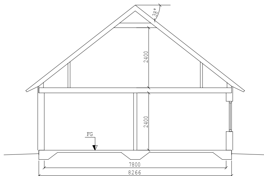
Sektion A-A
